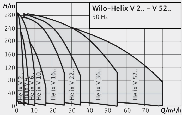
نمودار مشخصه پمپ‌های سری Helix V
